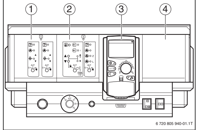
Res. 1 Modül donanımı
