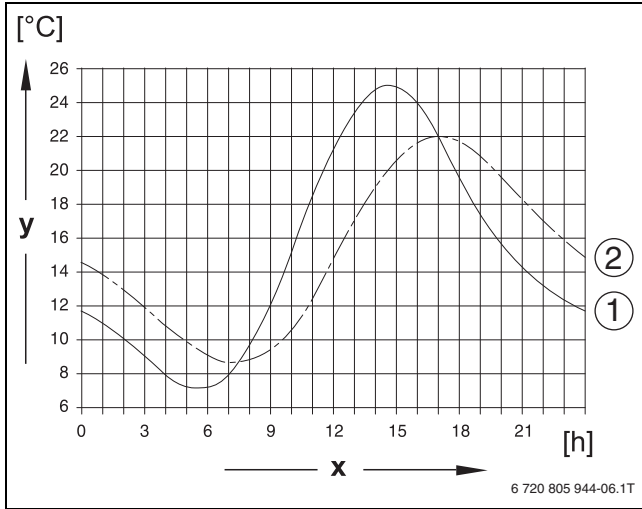
Res. 12 Güncel ve sönümlü dış hava sıcaklıklarının karşılaştırılması
