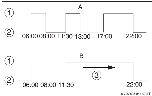
Res. 10 Isıtma evrelerinin birleştirilmesi
