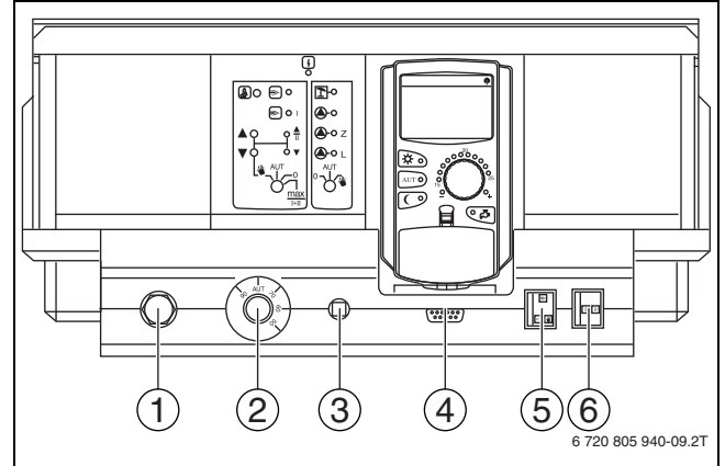
Res. 4 Kumanda paneli kumanda elemanları (Teslimat durumu)
